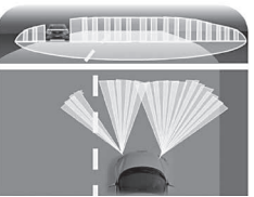
Deaktivierung einzelner LEDs, damit entgegenkommendes Fahrzeug nicht geblendet wird.
